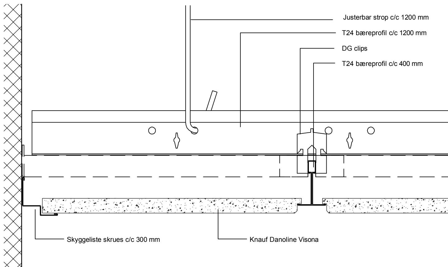
Snit A-A på tværs af profilretning
